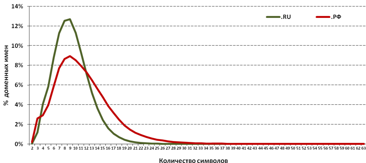
Рис.7. Длина доменных имен в доменах .RU и .RF (по состоянию на 31.12.2011)
